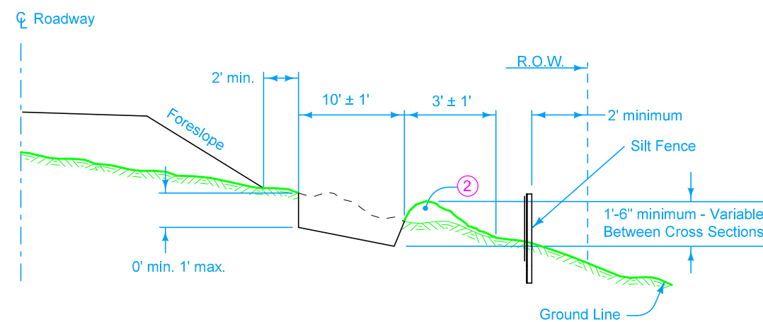
SILT DIKE
