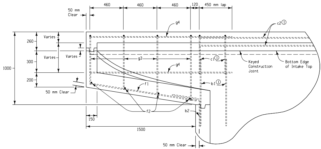
SECTION D-D
