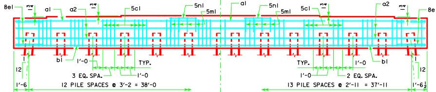
13 PILE BENT
