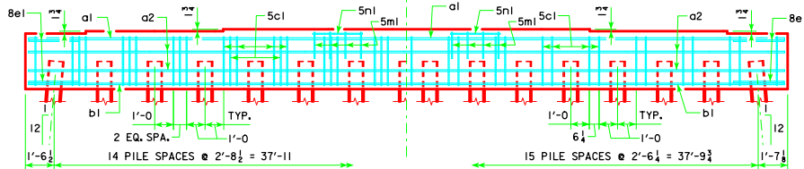
15 PILE BENT
