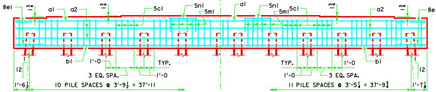
11 PILE BENT
