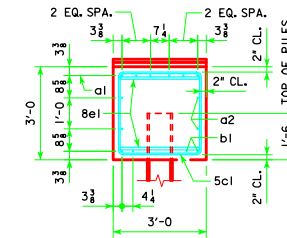
VIEW A-A
