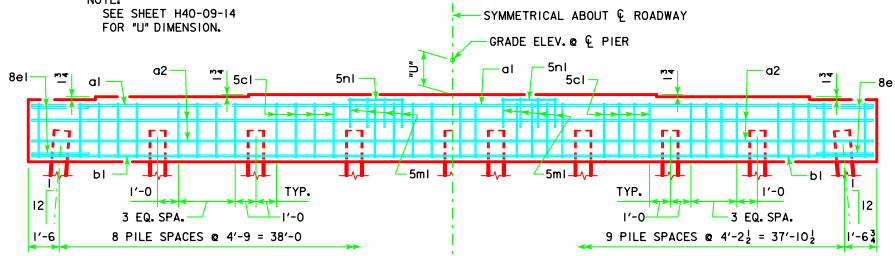
9 PILE BENT
