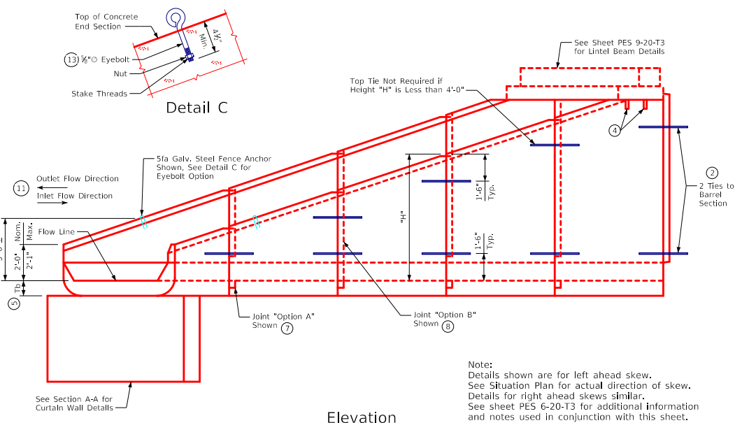
Elevation
