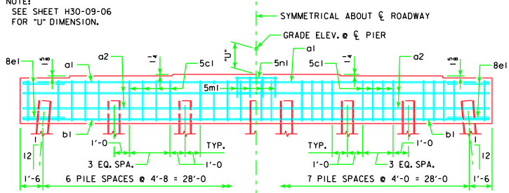
7 PILE BENT
