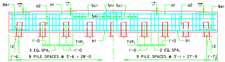
9 PILE BENT
