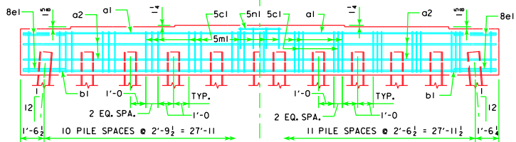
11 PILE BENT
