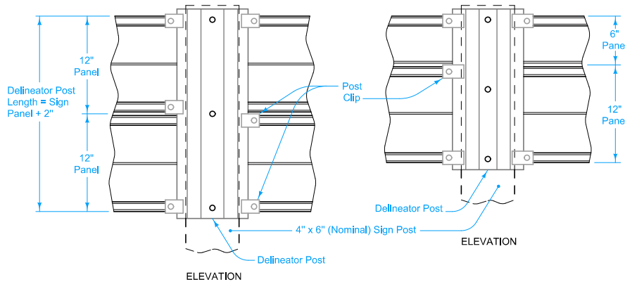
ELEVATION
