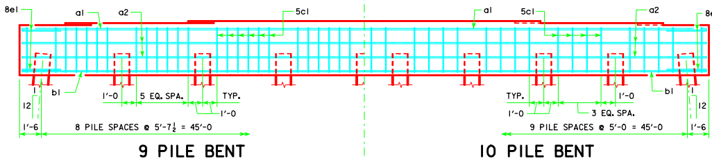
9 PILE BENT
