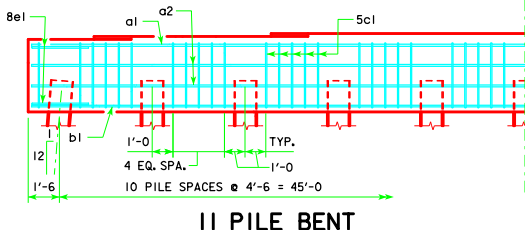
11 PILE BENT
