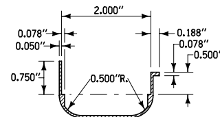
EDGE MOLDING
