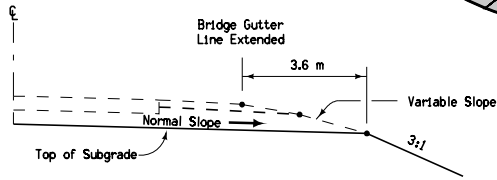
SECTION D-D
